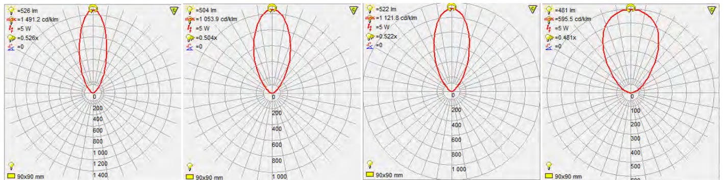
15° FWHM TIR
